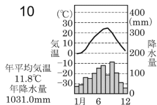
気候区分
