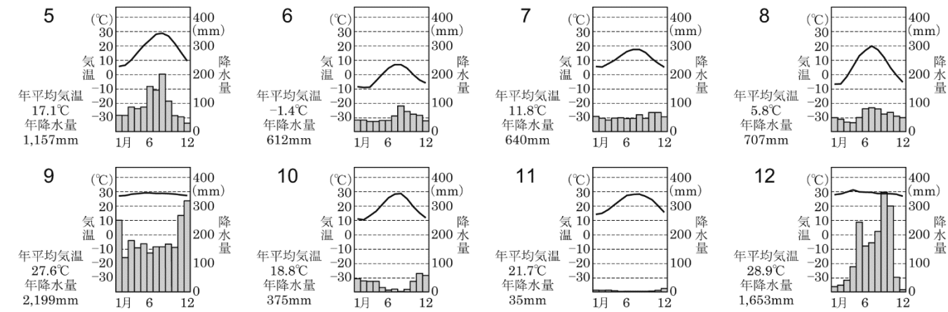
雨温図
