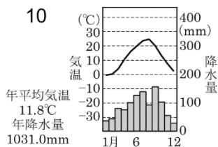
気候区分
