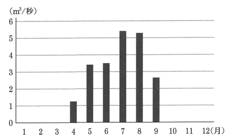
資料8 寺谷用水の月別利用水量（平均）
